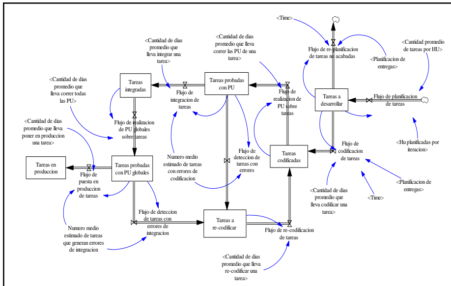
Fig. 6. Subsistema de Desarrollo de Tareas. (Fuente [13])
