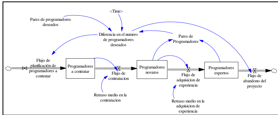
Fig. 1. Subsistema Recursos Humanos
