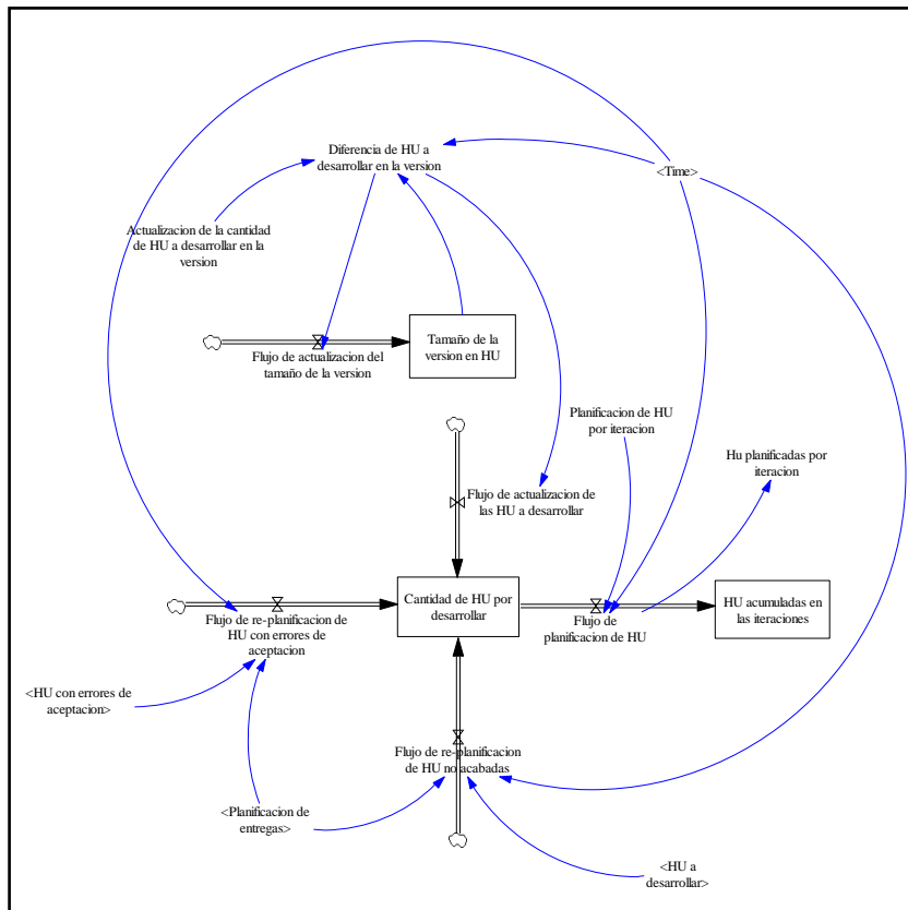
Fig. 5. Subsistema de Planificación
