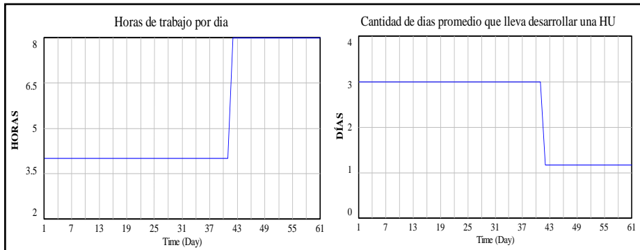
Fig. 10. Horas de Trabajo por Día y Cantidad de Días que lleva desarrollar una HU
