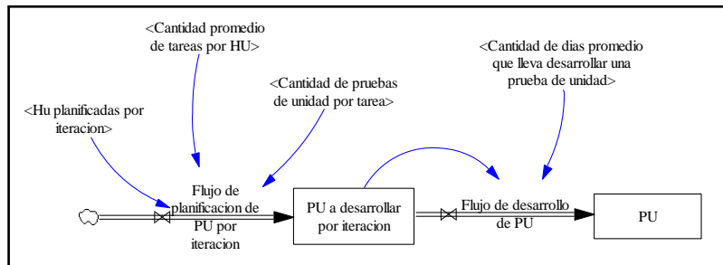
Fig. 3. Subsistema de Desarrollo de Pruebas de Unidad
