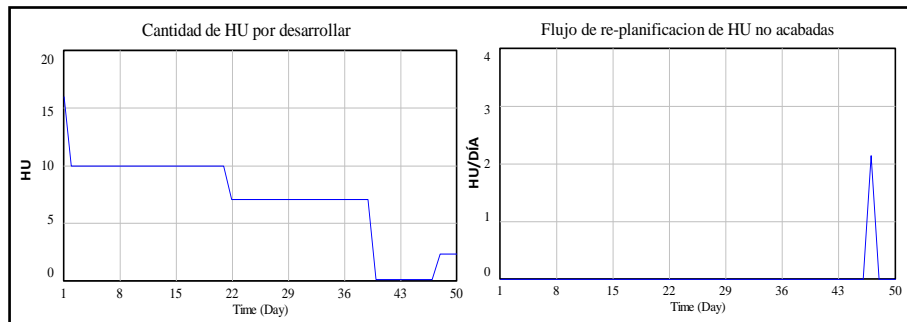
Fig. 8. Cantidad de HU por desarrollar y Re-planificación de HU no acabadas
