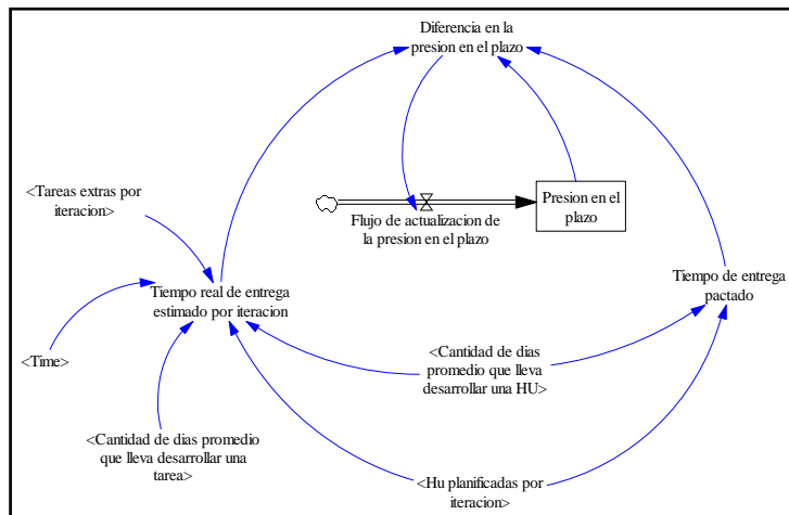
Fig. 4. Subsistema Presión en el Plazo
