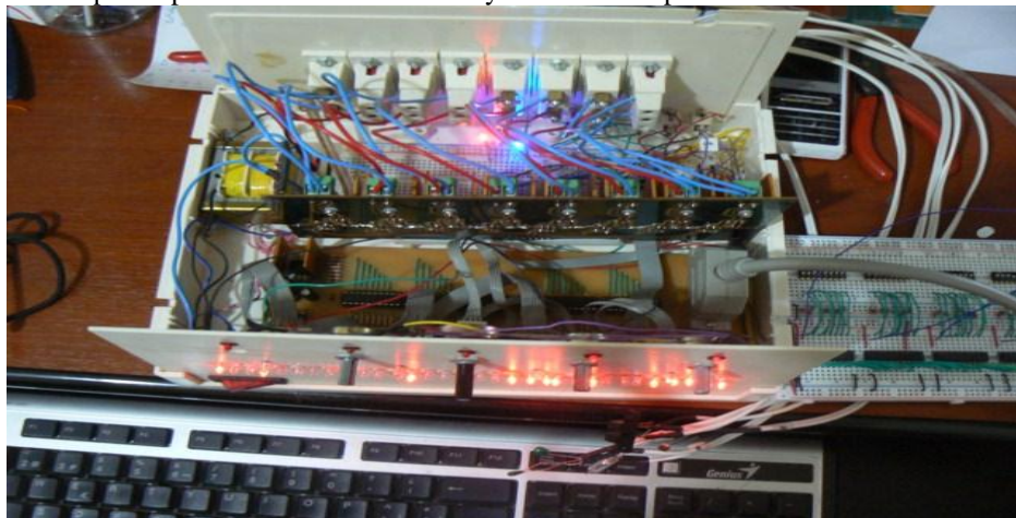
Fotografía 2. Ampliación del prototipo funcional de 5 entradas y 32 salidas.
